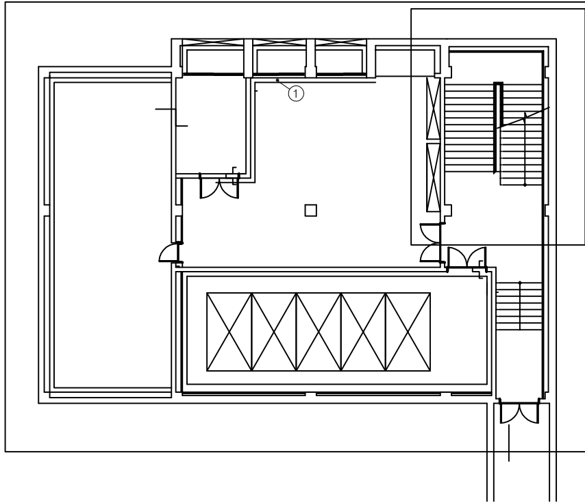
지하1층 평면
